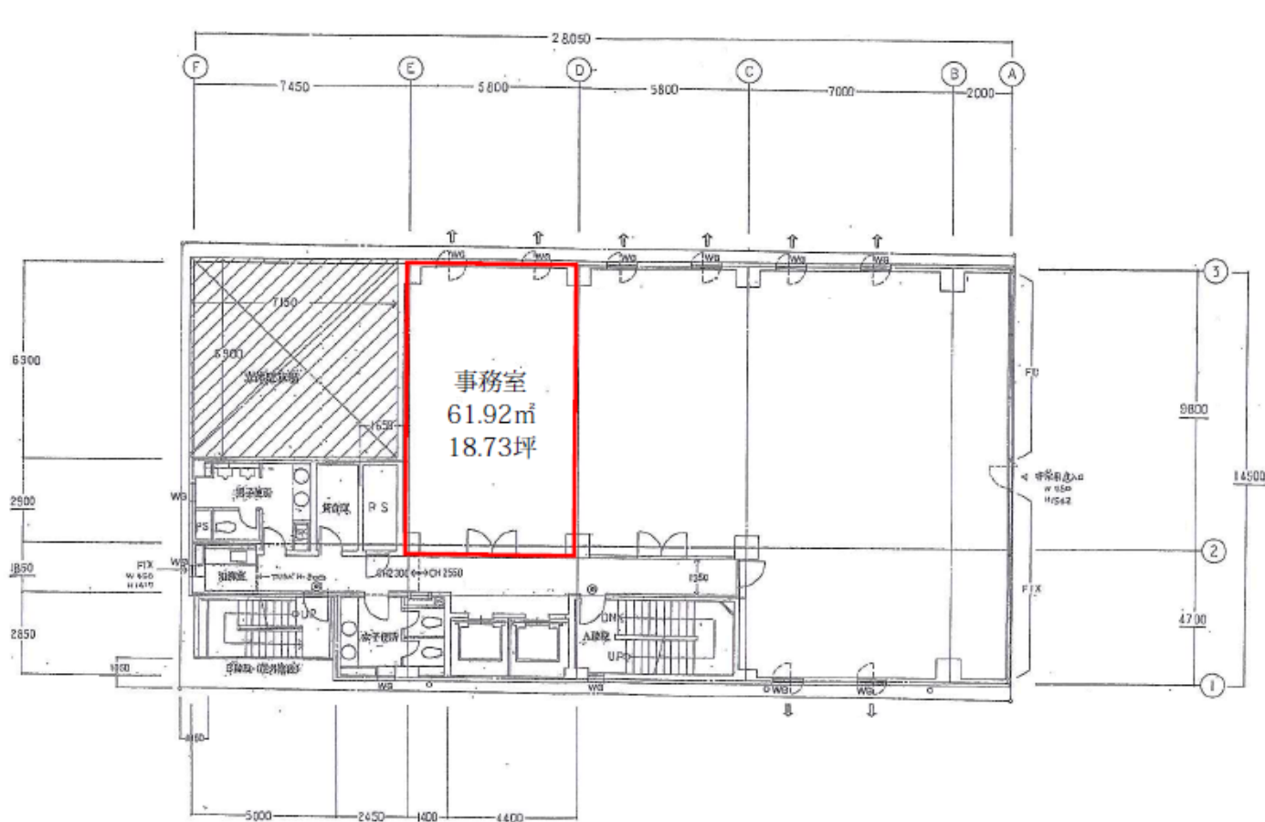
三同ビル錦 6F A号室 平面図
