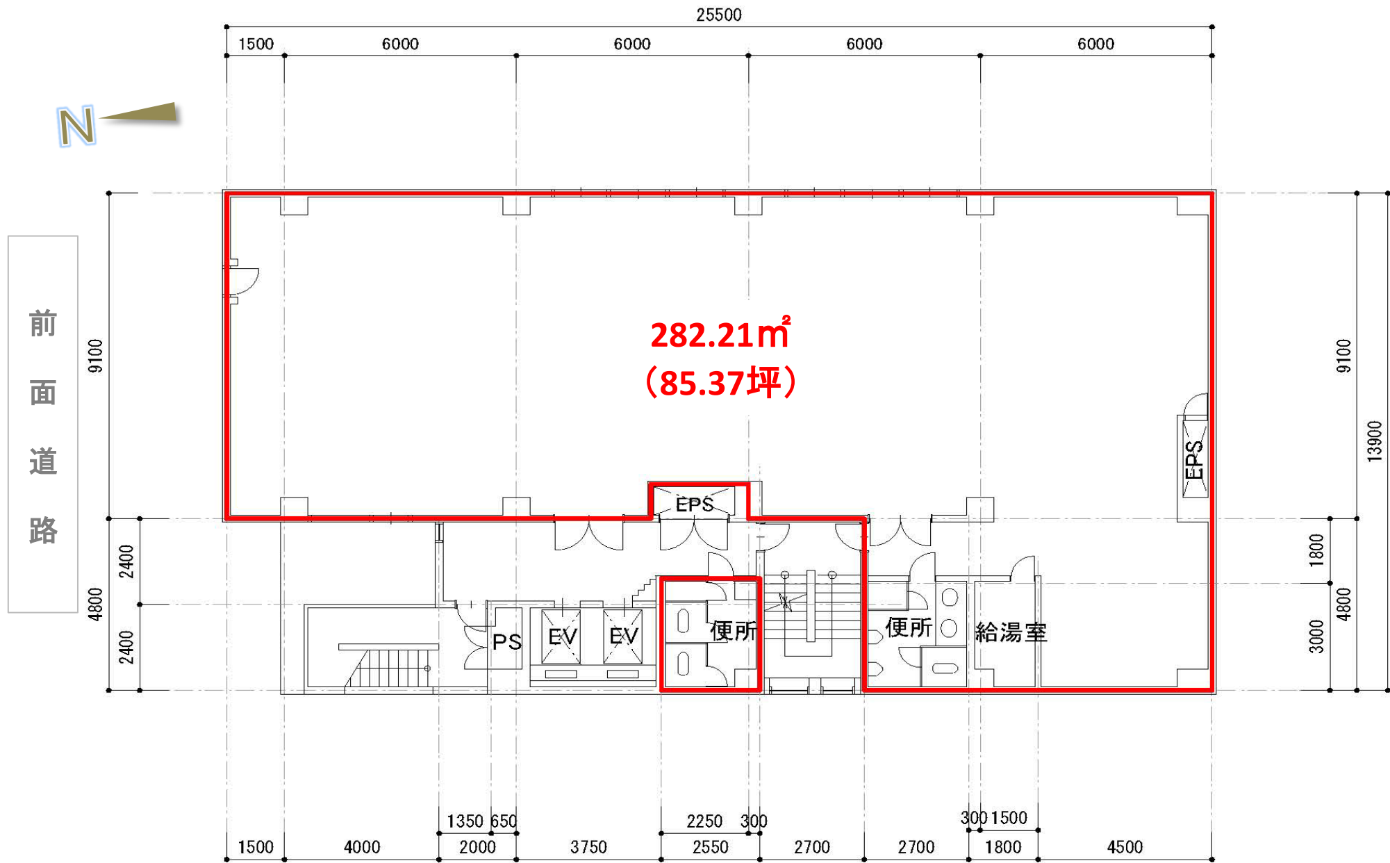
4階平面図
