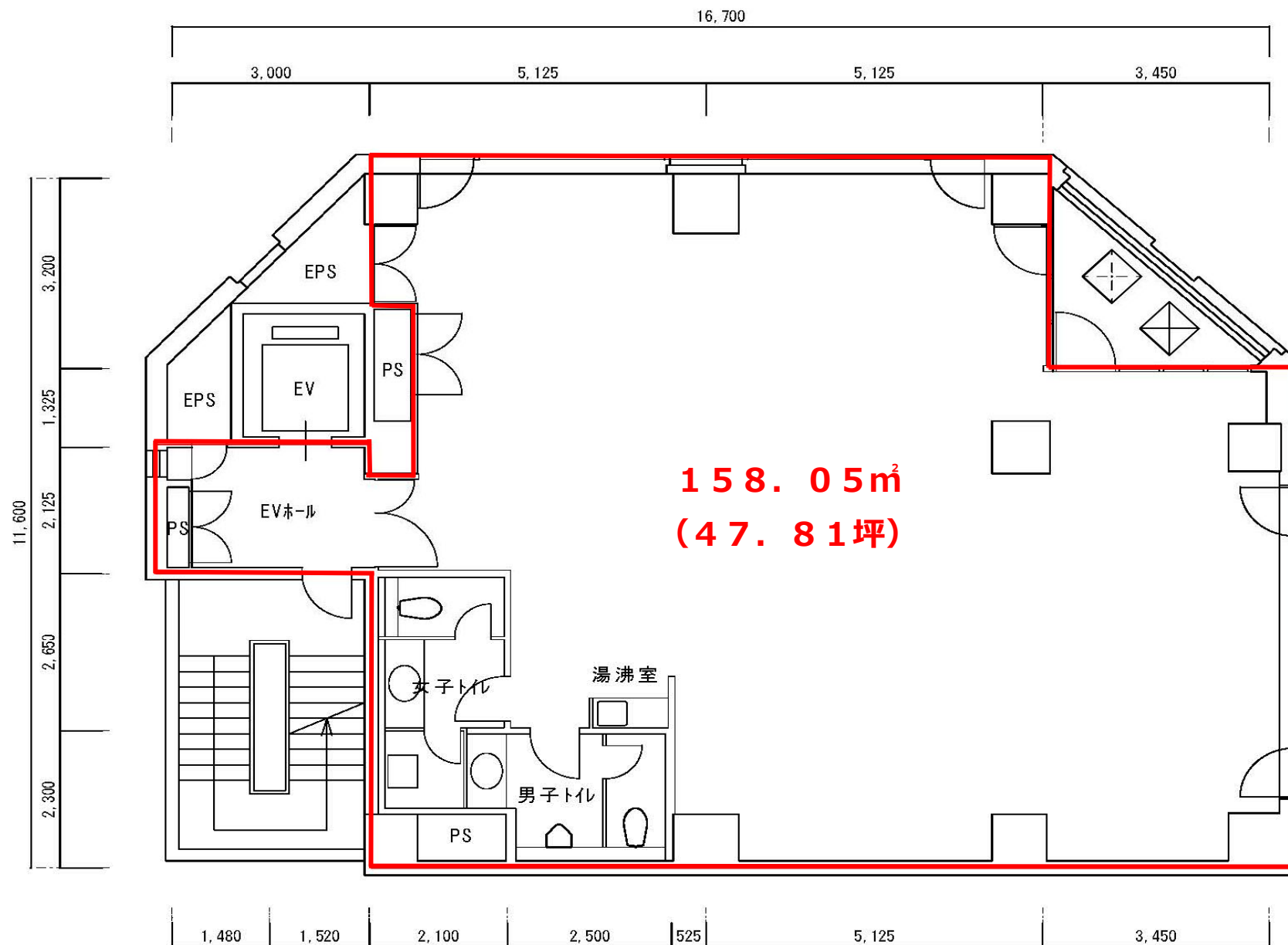
4階平面図
